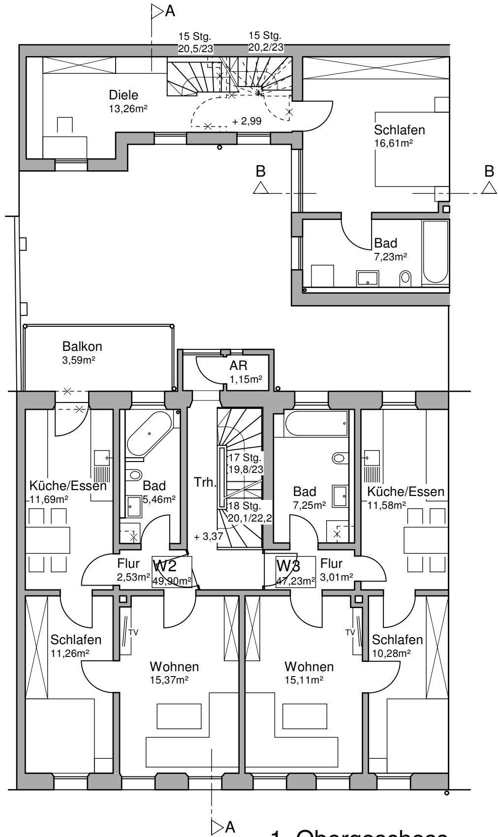
1. Obergeschoss
